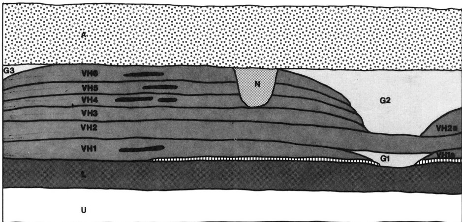
Skematisk opstilling af stratigrafien i Nicolajgade 8 set fra åsiden. Tegning: Børge H. Nielsen.
