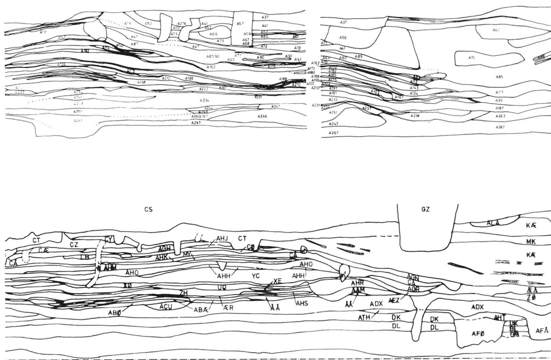
Fig. 7. Profilen gennem parcellen i Nicolajgade 8 (øverst) og udsnit af hovedprofilen i Kunstmuseets Have (nederst). Bemærk ligheden mellem de centralt placerede værkstedsaflejringer og parcelgrøfterne yderst til højre.
